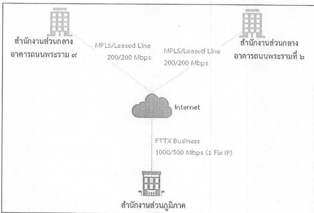
ภาพแสดงการเชื่อมโยงเครือข่ายสื่อสารข้อมูลและให้บริการอินเทอร์เน็ต
