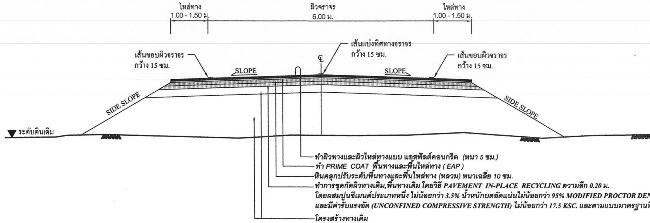
รูปตัดตามขวางงานซ่อมสร้างผิวทางแอสฟัลต์คอนกรีต NOT TO SCALE
